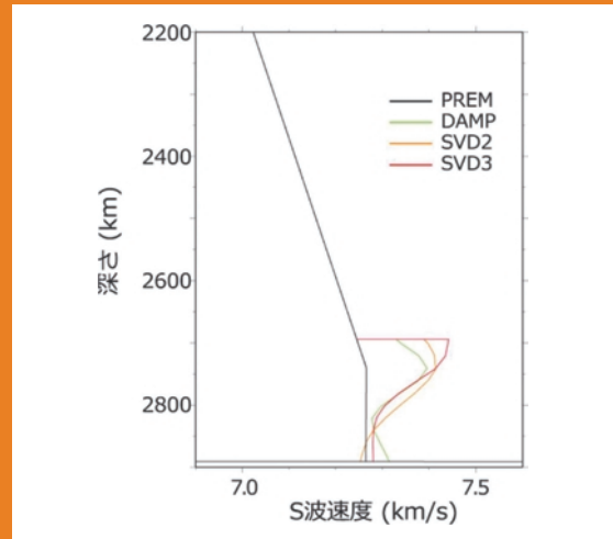
中米下のD"層のS波速度構造の標準モデル（PREM）と本研究が推定した3つのモデル。D"層上部では顕著な正の速度異常を示し、下半分では速度異常が小さいことがわかる。
