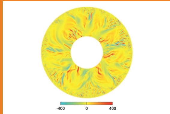
コア内部の熱対流のようす。赤道面上の流れの動径成分を色であらわしている。値は磁気レイノルズ数。内側の円は固体の内核の断面。はげしい乱流による電磁誘導によって電流が生成する。
